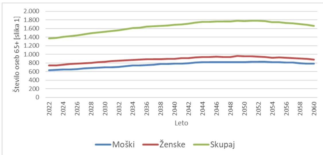
Slika 3.71 [slika 1]: Projekcije števila prebivalcev 65+ v občini Brda za obdobje od leta 2023 do leta 2060 (scenarij brez selitev – NMGR)
