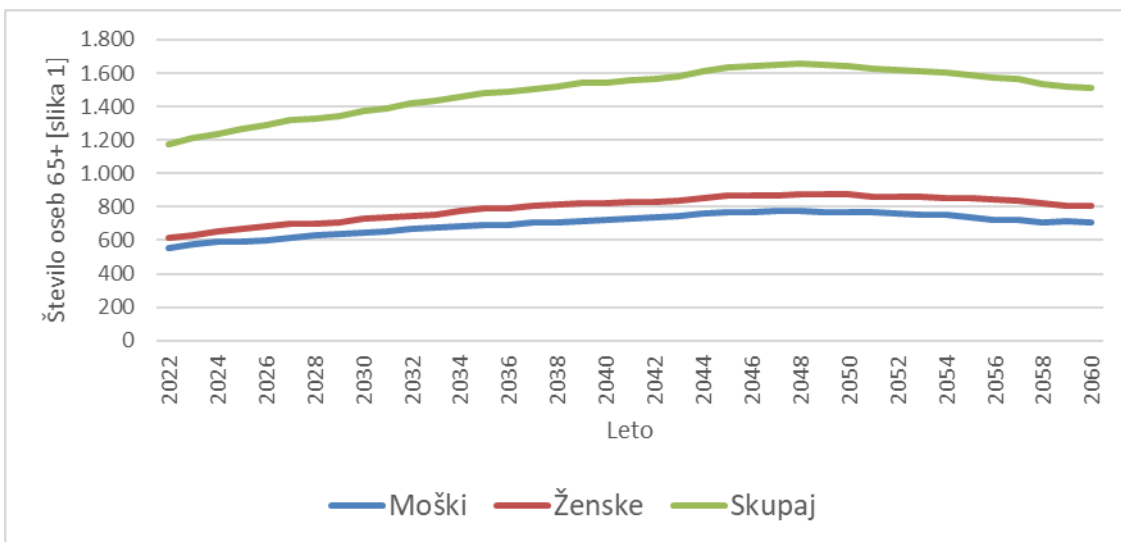
Slika 3.78 [slika 1]: Projekcije števila prebivalcev 65+ v občini Miren - Kostanjevica za obdobje od leta 2023 do leta 2060 (scenarij brez selitev – NMGR)
