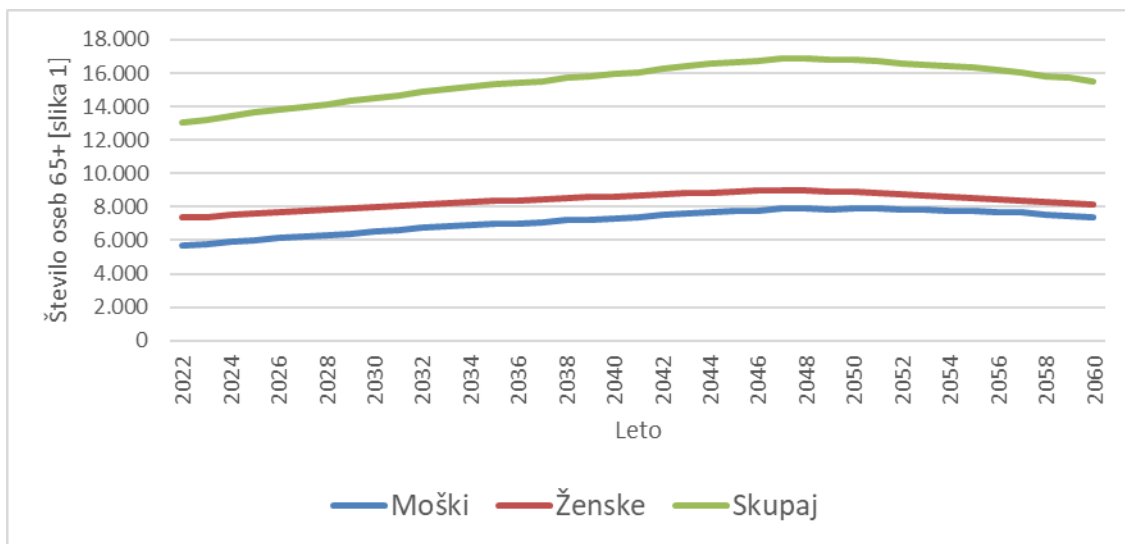
Slika 3.64 [slika 1]: Projekcije števila prebivalcev 65+ v LAS V objemu sonca za obdobje od leta 2023 do leta 2060 (scenarij brez selitev – NMGR)
