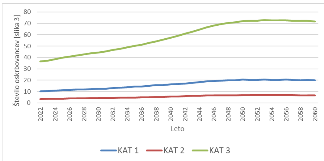
Slika 3.31 [slika 3]: Projekcije oskrbovancev v institucionalni oskrbi (DSO) po kategorijah zdravstvene nege v občini Kobarid do leta 2060 (scenarij brez selitev – NMGR)
