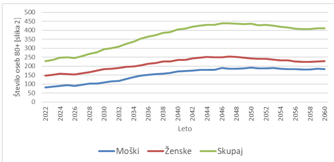
Slika 3.16 [slika 2]: Projekcije števila prebivalcev 80+ v občini Bovec za obdobje od leta 2023 do leta 2060 (scenarij brez selitev – NMGR)
