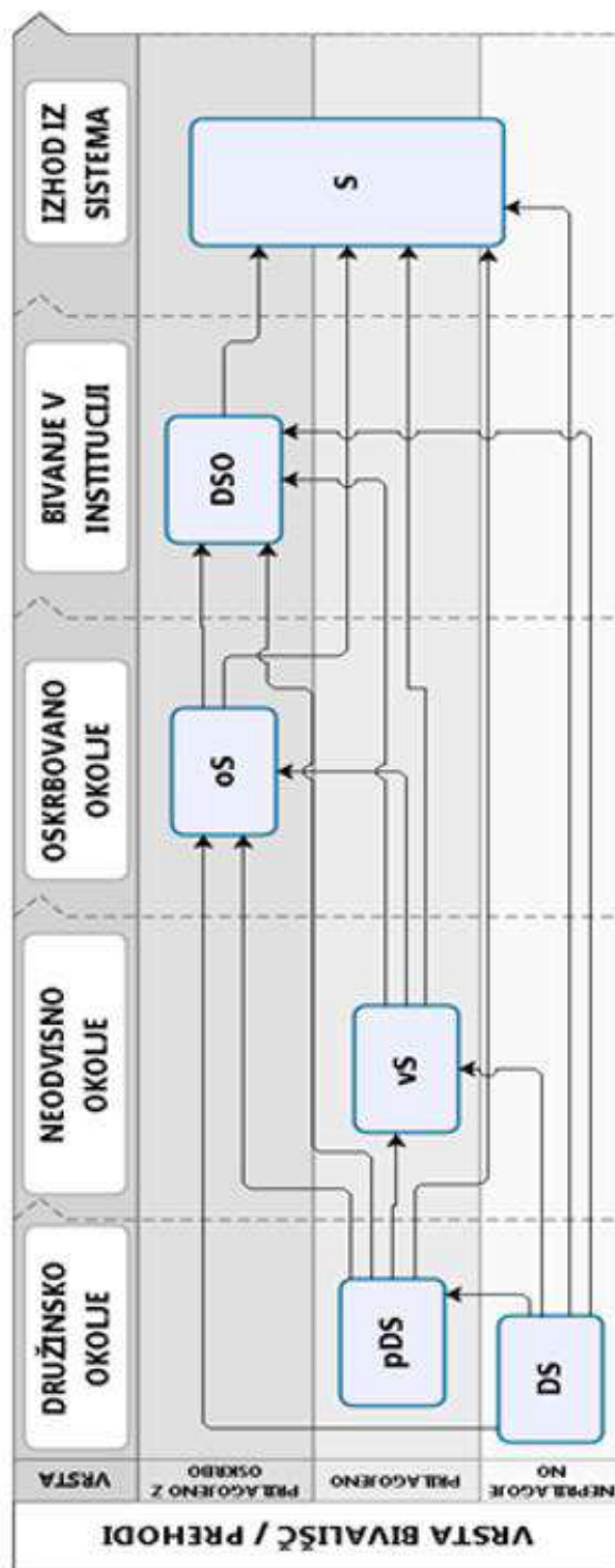
Slika 1.9: Diagram selitev med različnimi tipi bivališč starostnikov: iz lastnega doma do doma starejših občanov (DSO) v okviru modela mnogoterih pojemanj
